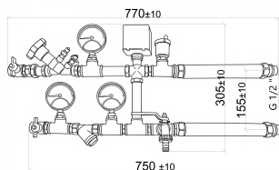
Размеры водяной обвязки для фанкойла
